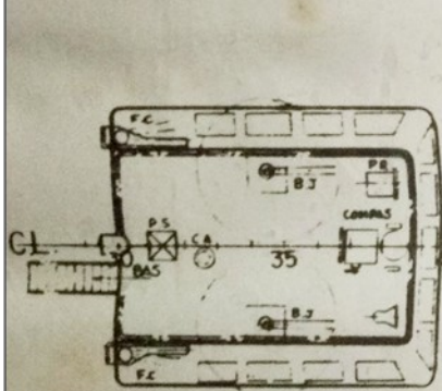
SOMMET DE LA TIMONERIE (HUNE) WHEEL HOUSE TOP
